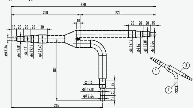
Жидкостная труба
