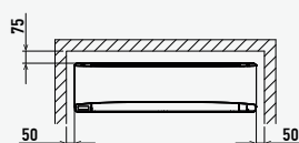
Минимальные требования к пространству для установки
