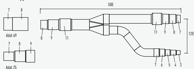
Газовая труба
