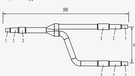
Жидкостная труба
