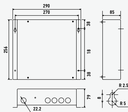
АДАПТЕР СВЯЗИ (CZ-CFUNC2)
