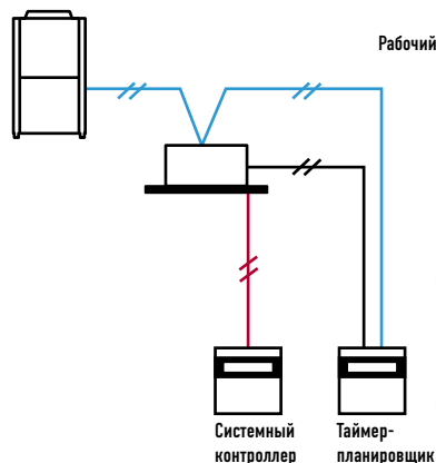
Пример подключения 1 (питание от внутреннего блока)
