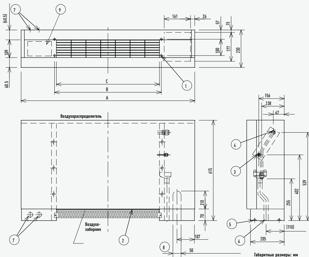
Габаритные размеры: мм
