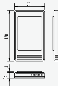
Упрощенный пульт ДУ (CZ-RE2C2) Датчик для ПДУ (CZ-CSRC2)
