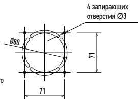
Размер соединительного порта воздуховода (приточного воздуха)
