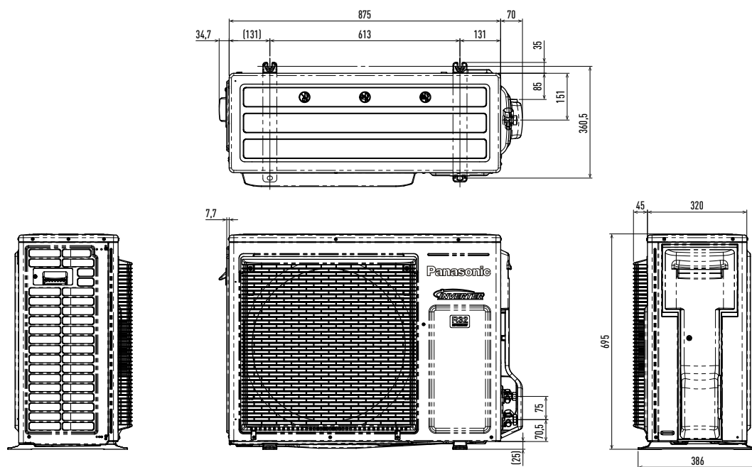
Наружный блок PACi R32: маленький, 1 вентилятор
