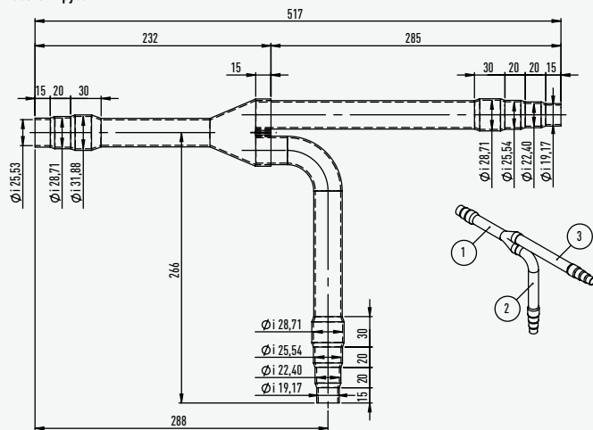
Газовая труба
