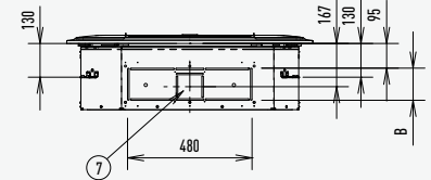
ВИД В РАЗРЕЗЕ
