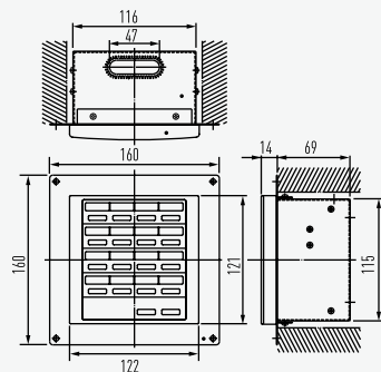
Регулятор ВКЛ / ВЫКЛ (CZ-ANC2)
