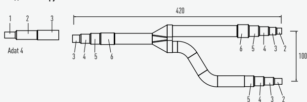
Жидкостная труба
