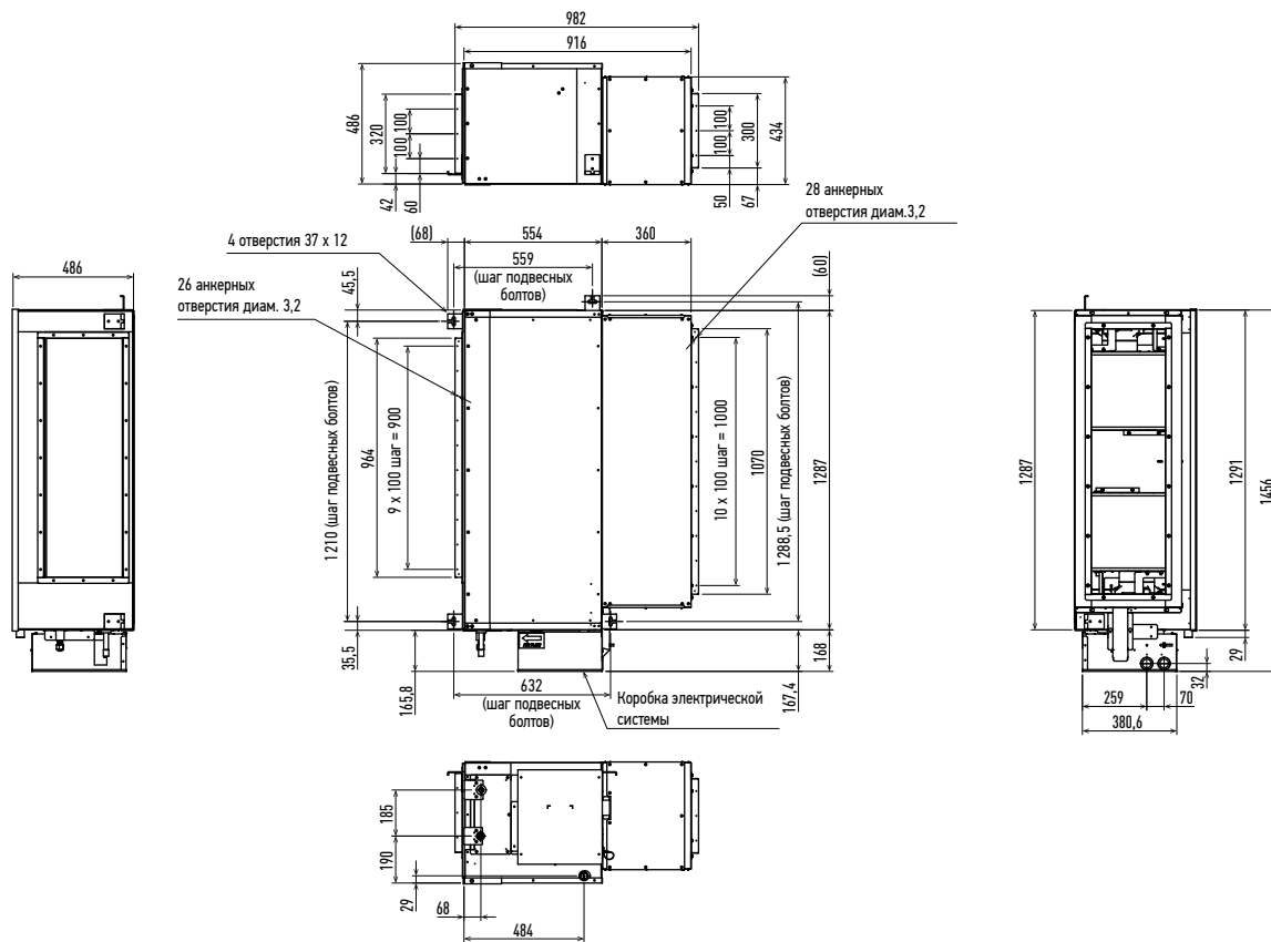
Блок высокого статического давления и скрытого монтажа PACi 20,00-25,00 кВт
