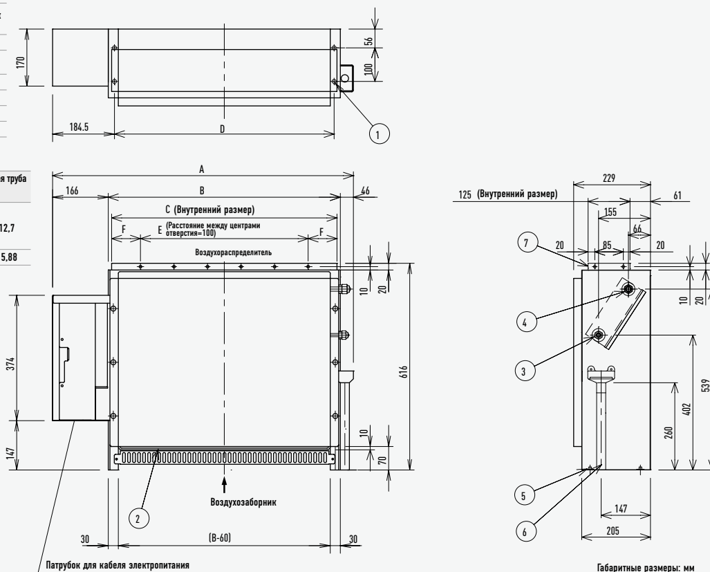
Габаритные размеры: мм
