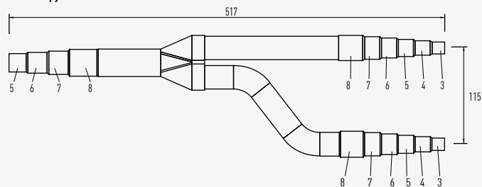
Газовая труба
