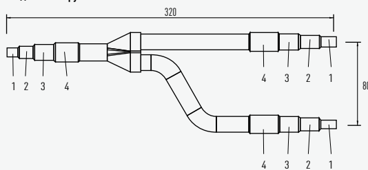
Жидкостная труба
