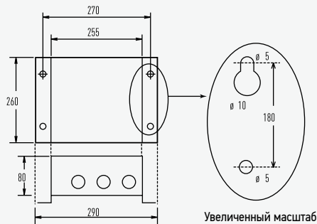
КОНТРОЛЛЕР ВВОДА / ВЫВОДА SERI-PARA I / O ДЛЯ ВНЕШНЕГО БЛОКА (CZ-SAPBC2)
