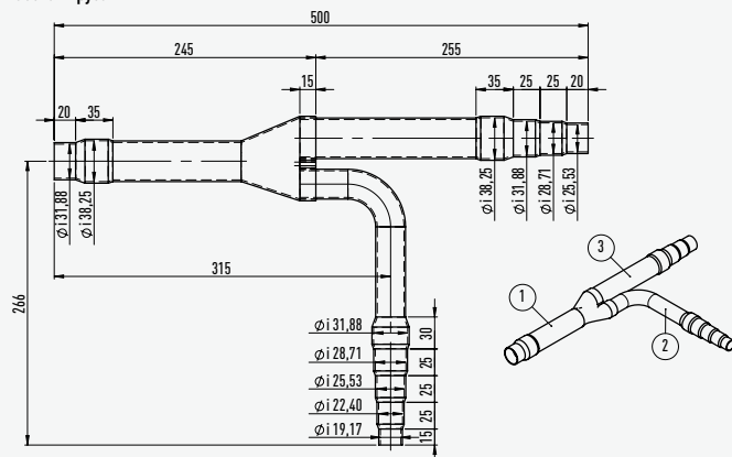
Газовая труба
